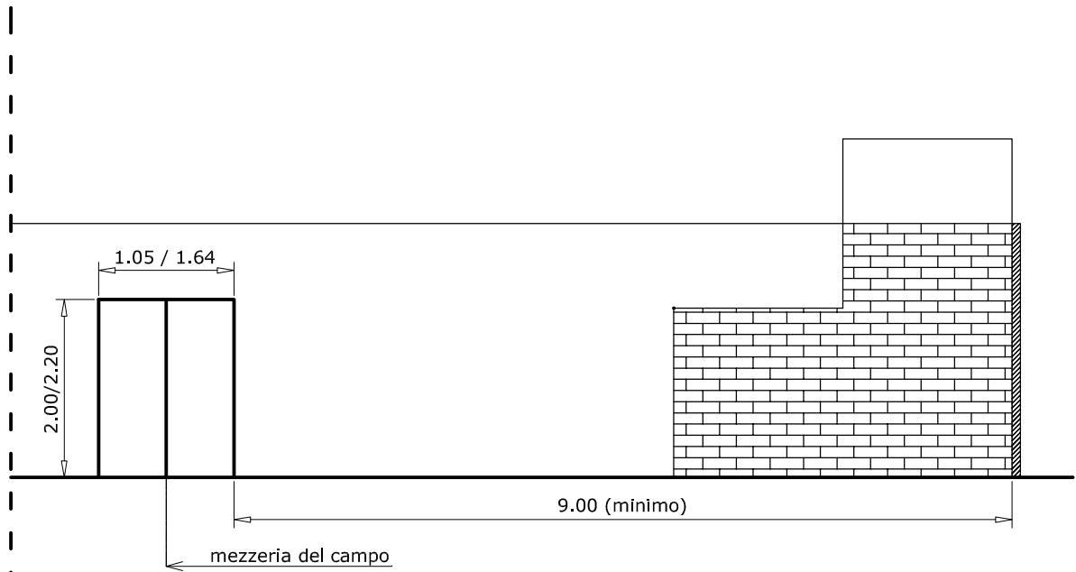
CAMPO CON PARETI IN MURATURA
