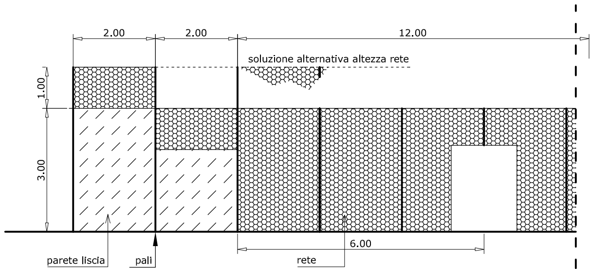
PROSPETTO LATERALE (misure in metri)
