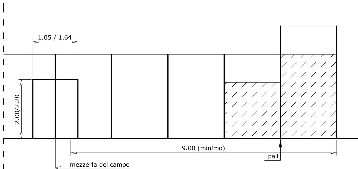
CAMPO CON RECINZIONE A PALI
