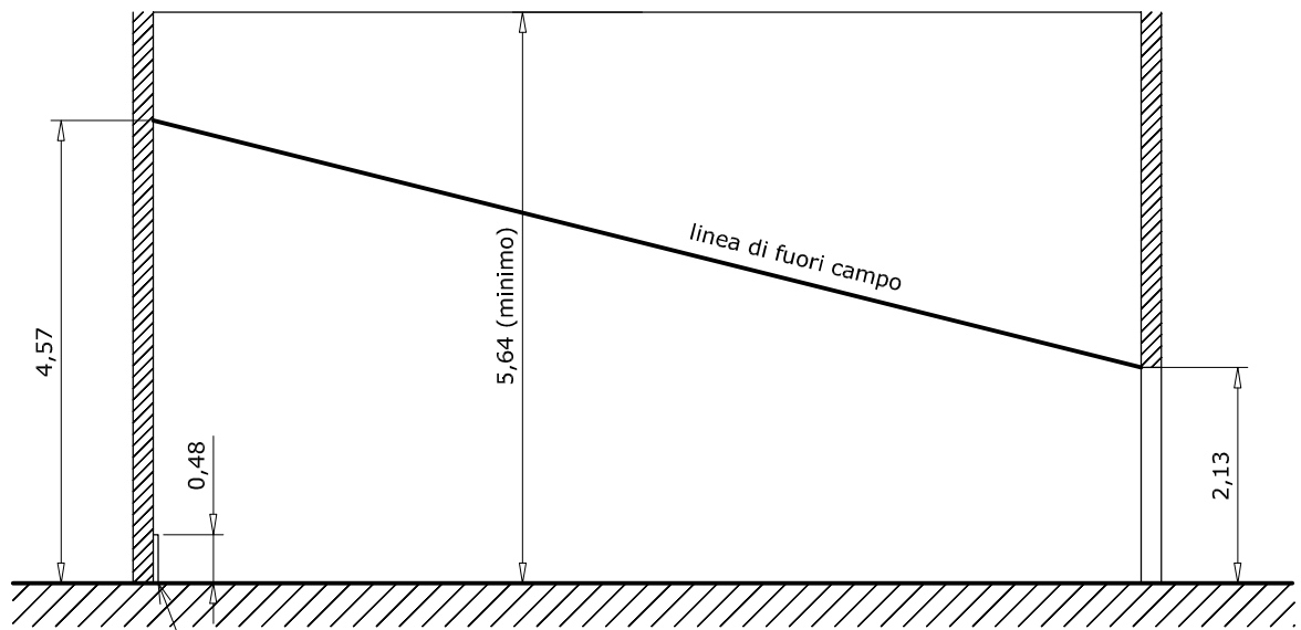
PARETE LATERALE
