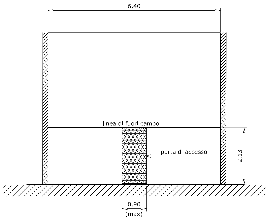
PARETE POSTERIORE
