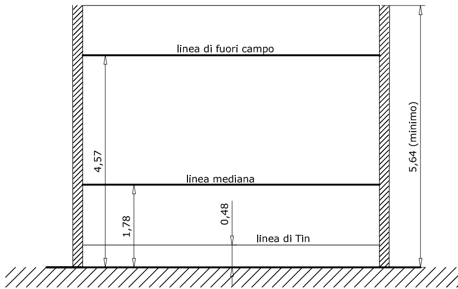
PARETE FRONTALE
