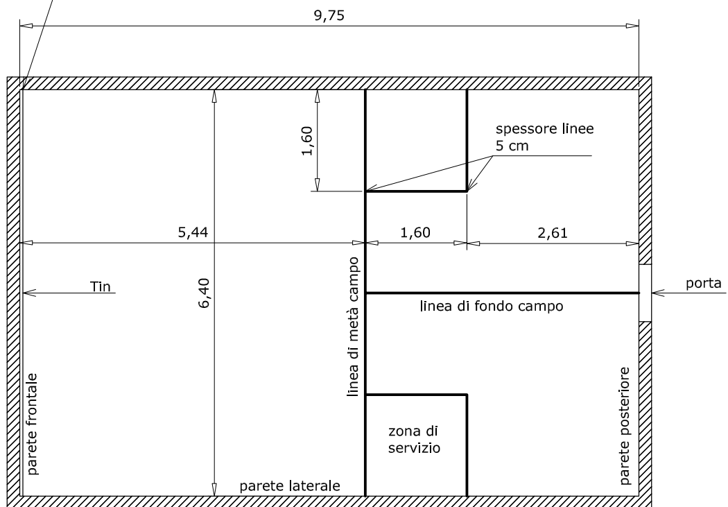
PIANTA
