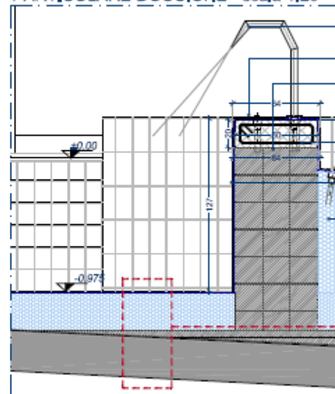
PARTICOLARE DOCCIONE - scala 1:20
