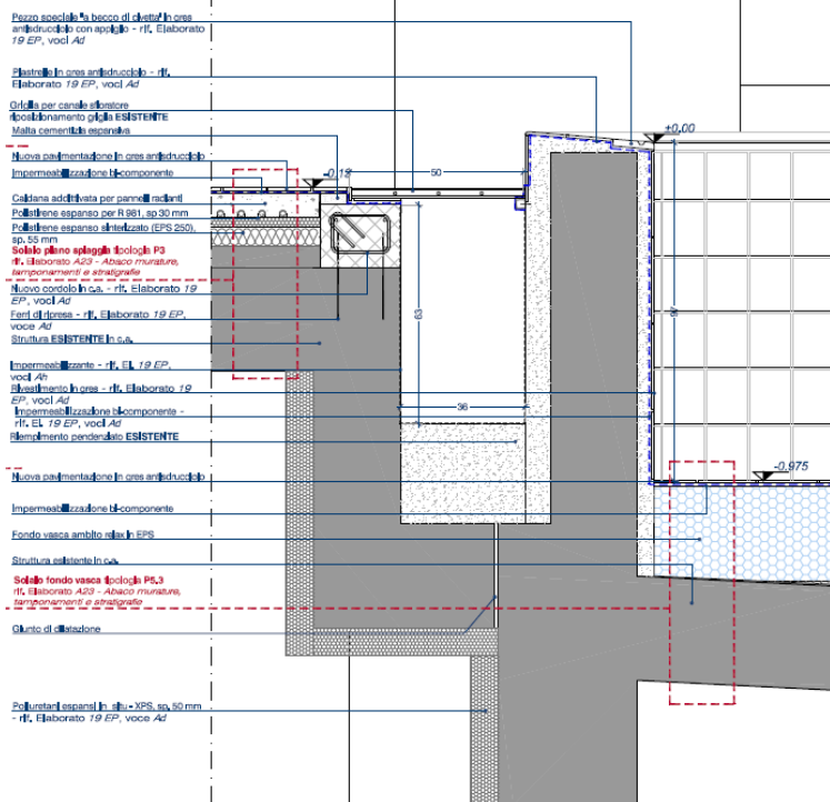
Dettaglio n° 5 Stralcio sezione B-B - scala 1:10
