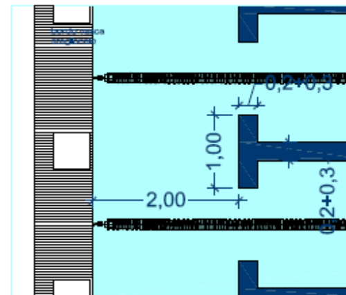
PIANTA SEGNAZIONE IN PROSSIMITA' DELLA TESTATA
