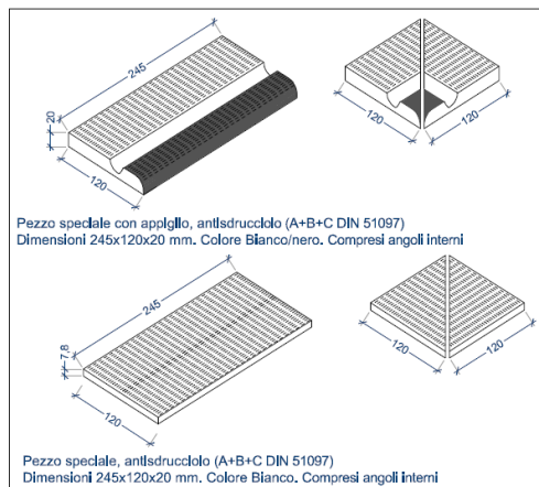
PROSPETTO SEGNAZIONE IN TESTATA
