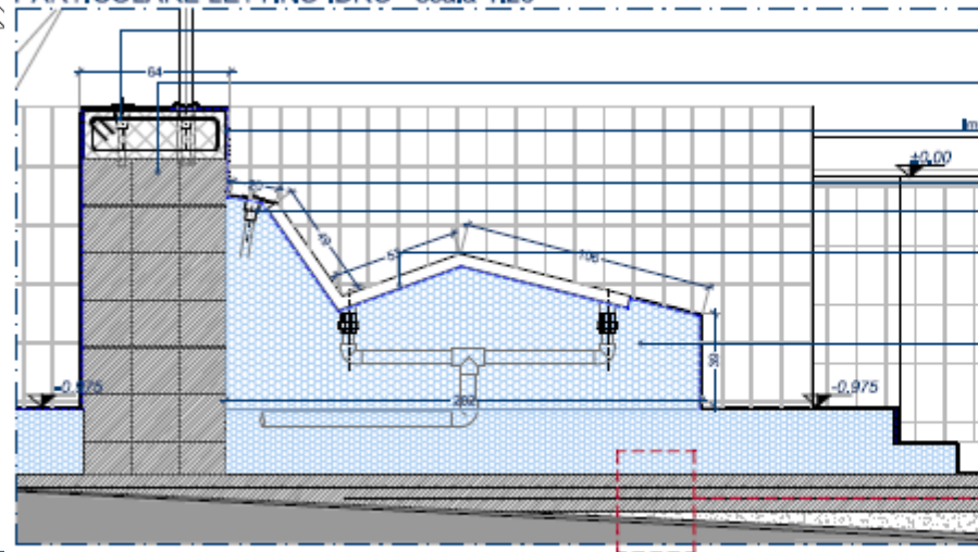
PARTICOLARE LETTINO IDRO - scala 1:20
